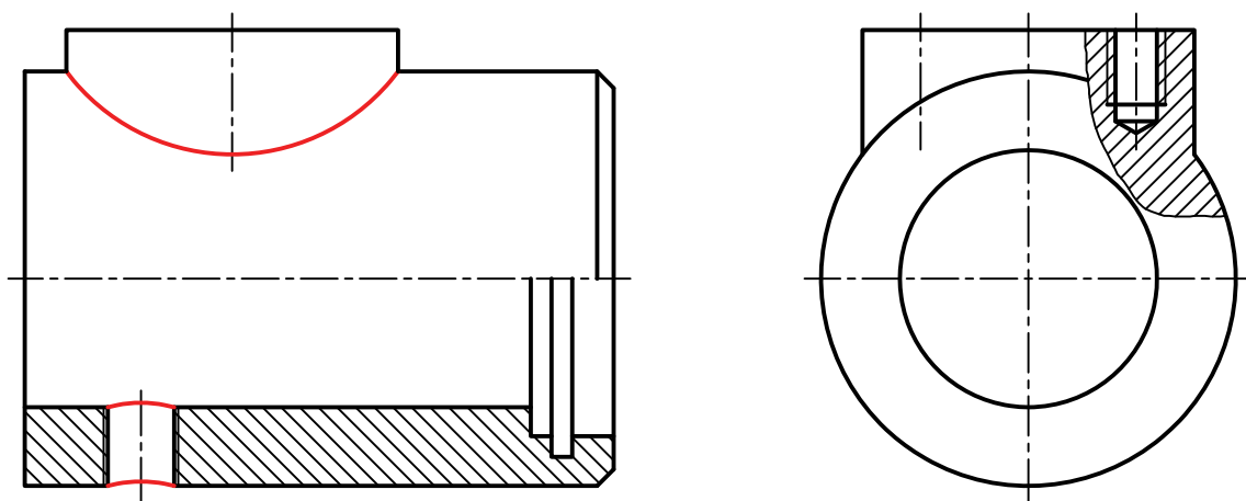
شکل ۱۵-۲۶- بدنه ضامن
