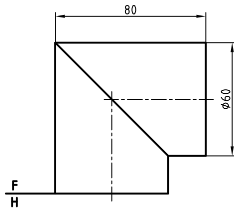
شکل ۱۶-۳۵- زانو
